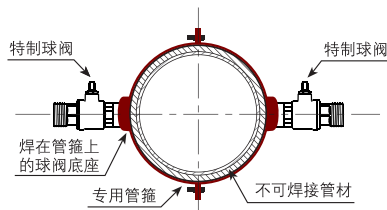
管箍固定球阀底座
