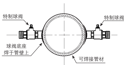
焊接固定球阀底座
