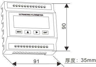
安装图
