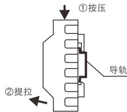
拆卸图
